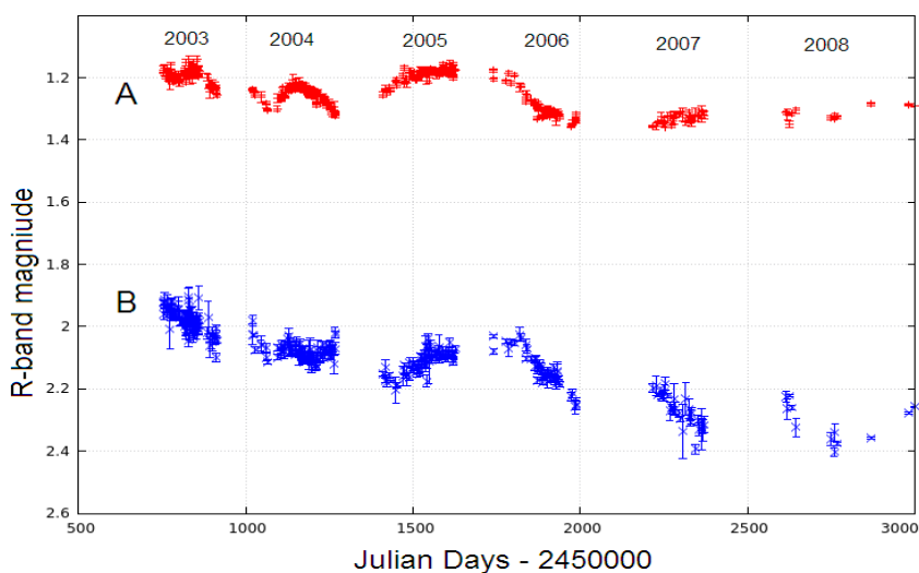
5-расм. SBS 1520+530 ГЛКнинг A ва B компонентлари равшанлик эгри чизиқлари.
