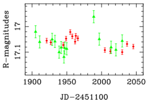
3-расм. А компоненти ҳамда вақт ва равшанлиги бўйича силжиган В нинг равшанлик эгри чизиқлари.
