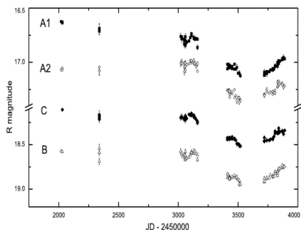
8-расм. PG 1115+080 ГЛК компонентларининг равшанлик эгри чизиқлари.
