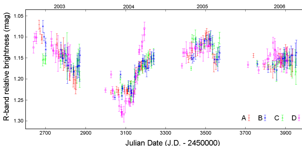
10-расм. Кечикиш вақтлари ҳисобга олинган ҳолда Н1413+117 ГЛКнинг А, В, С, D линзаланган компонентларининг R – филътрадаги равшанлик эгри чизиқлари.
